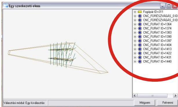
Integrált gépi lista egy fadarab nézeténél
